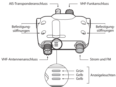
Abbildung 2 AIS-Antennenweiche-Übersicht
