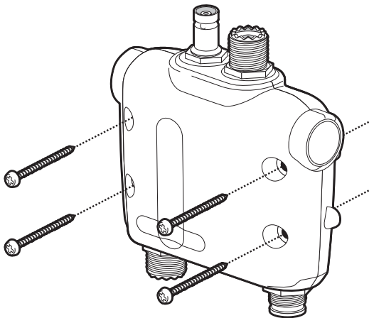
Abbildung 5 AIS-Antennenweiche Montage
