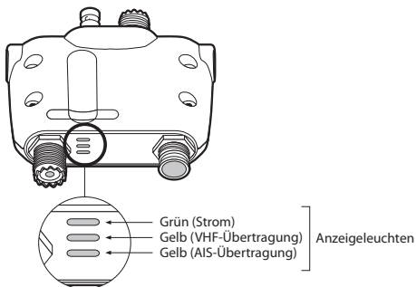
Abbildung 10 Anzeigeposition des AIS-Antennenweiche-Geräts
