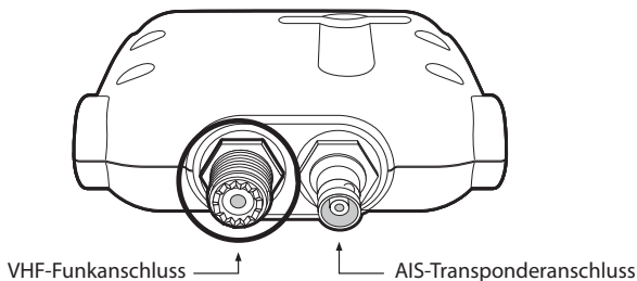
Abbildung 7 Position des VHF-Funkgerät-Anschlusses
