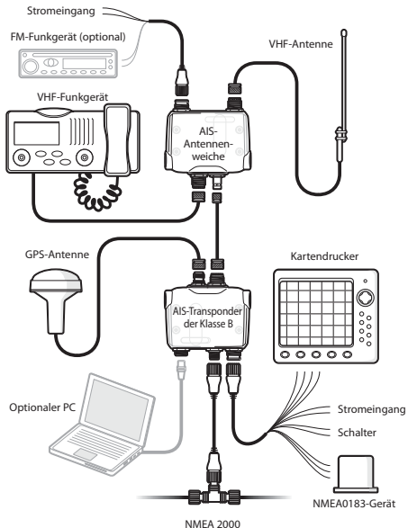
Abbildung 3 Typische Installationskonfiguration
