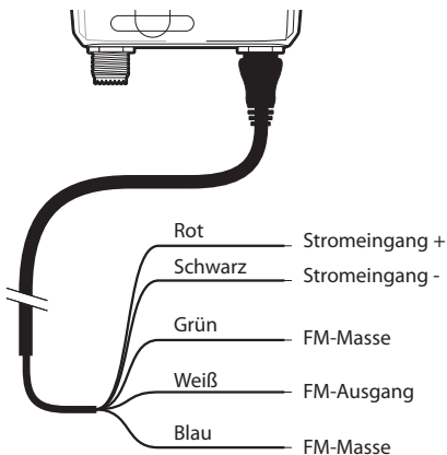
Abbildung 9 Anschluss der Stromversorgung und des optionalen FM-Ausgangs
