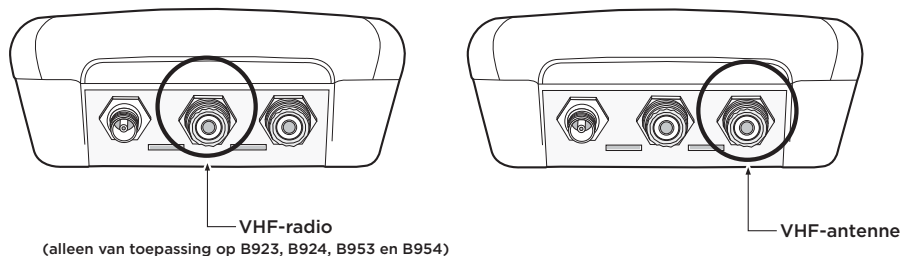
Figuur 6 Positie van de VHF-antenne-aansluiting
