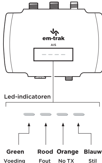
Figuur 20 Led-indicatorlocatie op de AIS transceiver-eenheid
