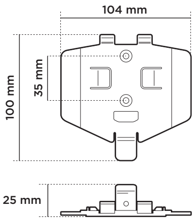
Figuur 10 Afmetingen van de AIS transceiver
