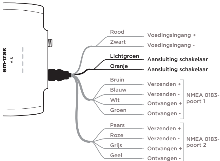
Figuur 21 Een externe schakelaar aansluiten
