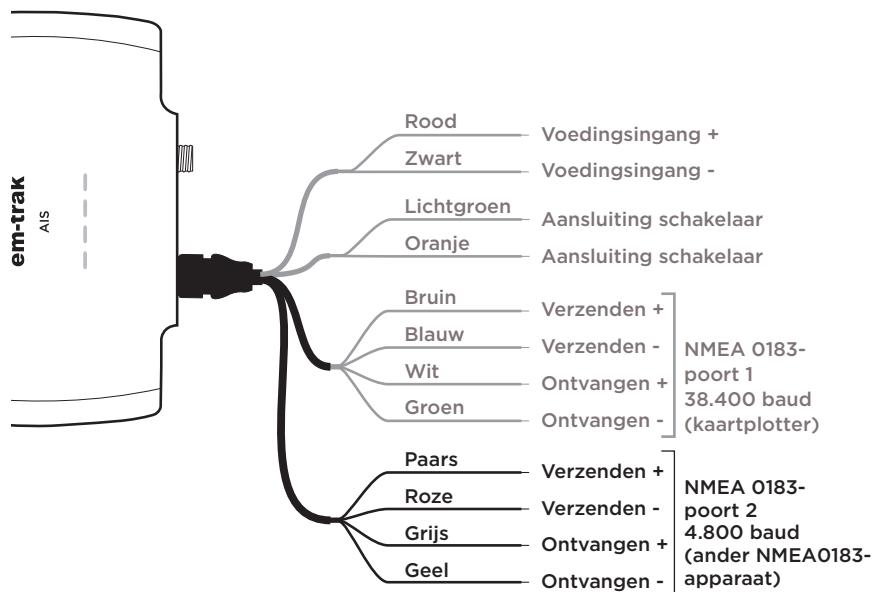
Figuur 18 Verbinding maken met uw NMEA 0183-sensor
