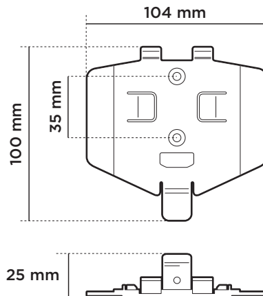
Figuur 2 Afmetingen van transceiver
