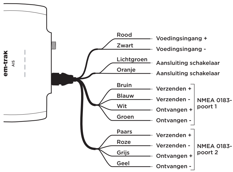
Figuur 8 Voedings- en gegevenskabel aangesloten
