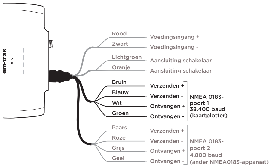
Figuur 17 Verbinding maken met uw kaartplotter
